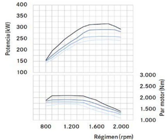
Curva de motor: OM 470 (290 kW)
